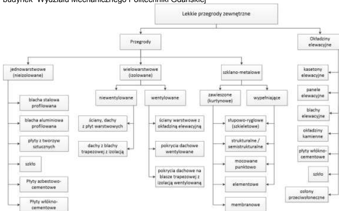
Rys. 3. Klasyfikacja lekkich przegród zewnętrznych
