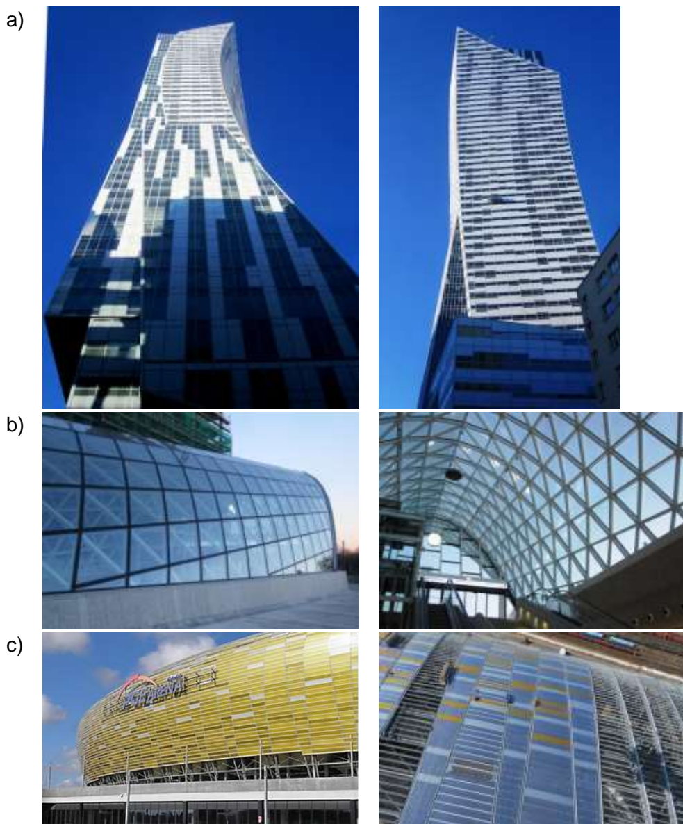
Rys. 1. Przykłady dowolnego kształtowania bryły obiektów z lekką obudową (fot. D. Kowalski) a) obiekt wysoki kubaturowy, b) przekrycie wejścia do pasażu podziemnego, c) fasada ścienna i przekrycie dachowe zadaszenia obiektu sportowego [4, 6, 7],
